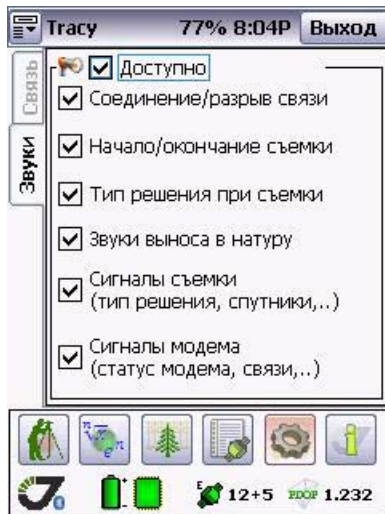
Рисунок 6-2. Закладка Звуки
