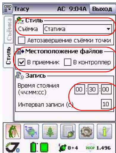
Рисунок 8-1. Закладка Стиль
