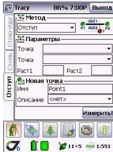
Рисунок 2-16. Закладка Отступ
