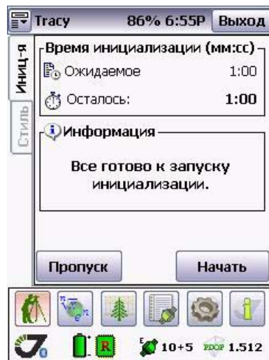
Рисунок 8-4. Закладка Инициализация
