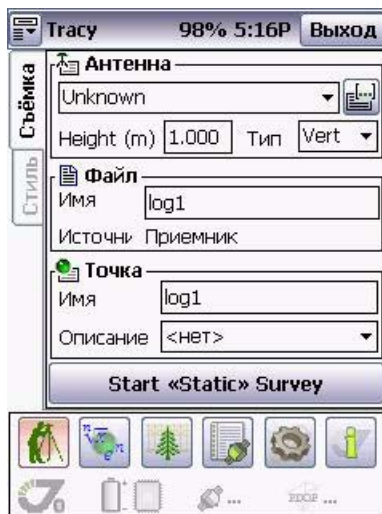
Рисунок 2-1. Закладка Съемка
