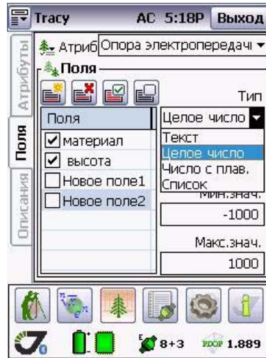
Рисунок 4-4. Поле Поля
