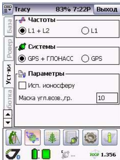
Рисунок 3-5. Закладка Установки
